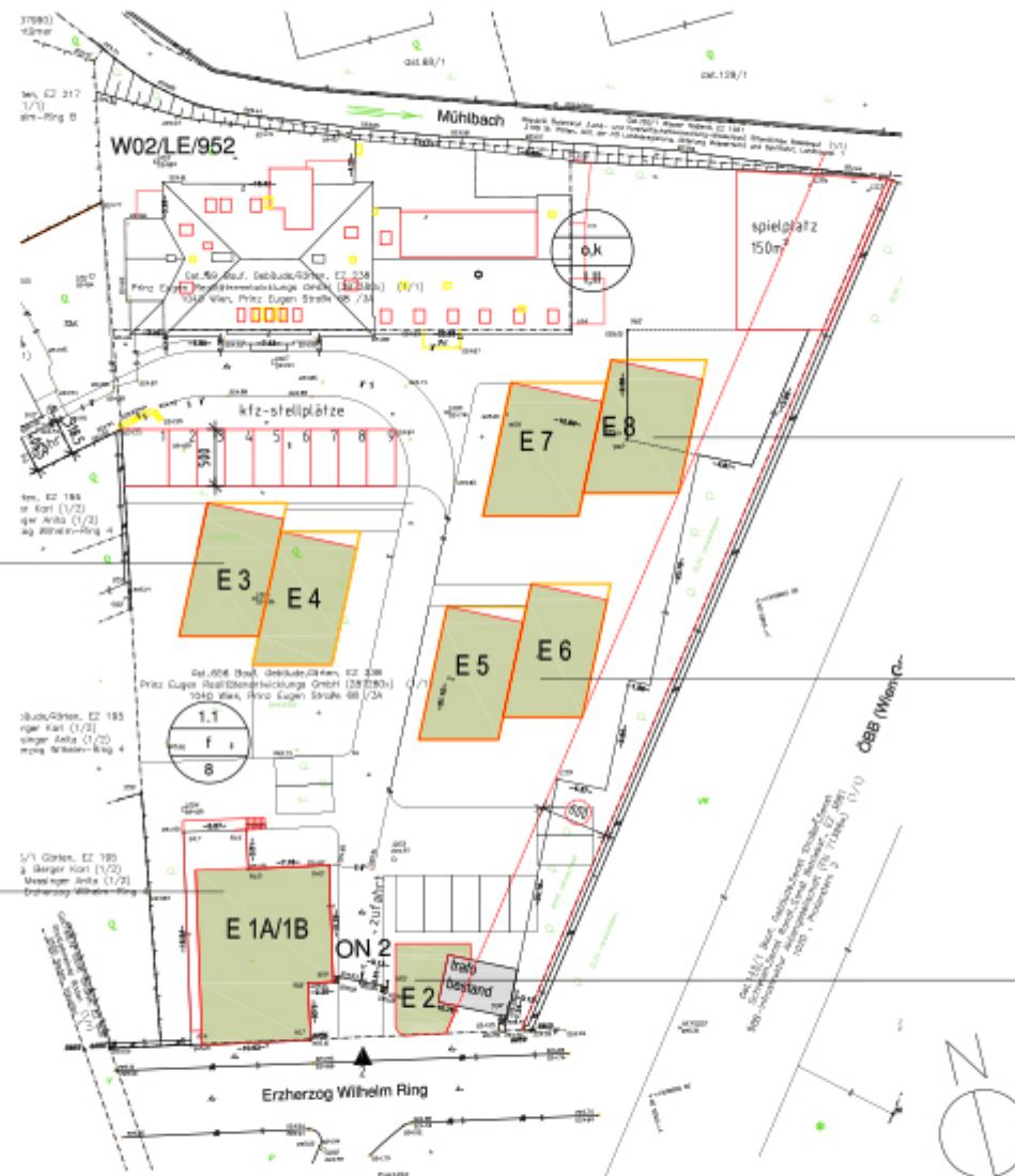
lageplan 1:500
